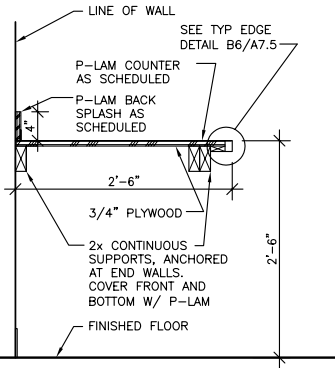
A4 A7.5 COUNTER SECTION 1" = 1'-0"
