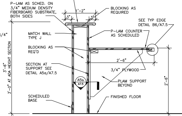
A5 A7.5 COUNTER SECTION 1" = 1'-0"
