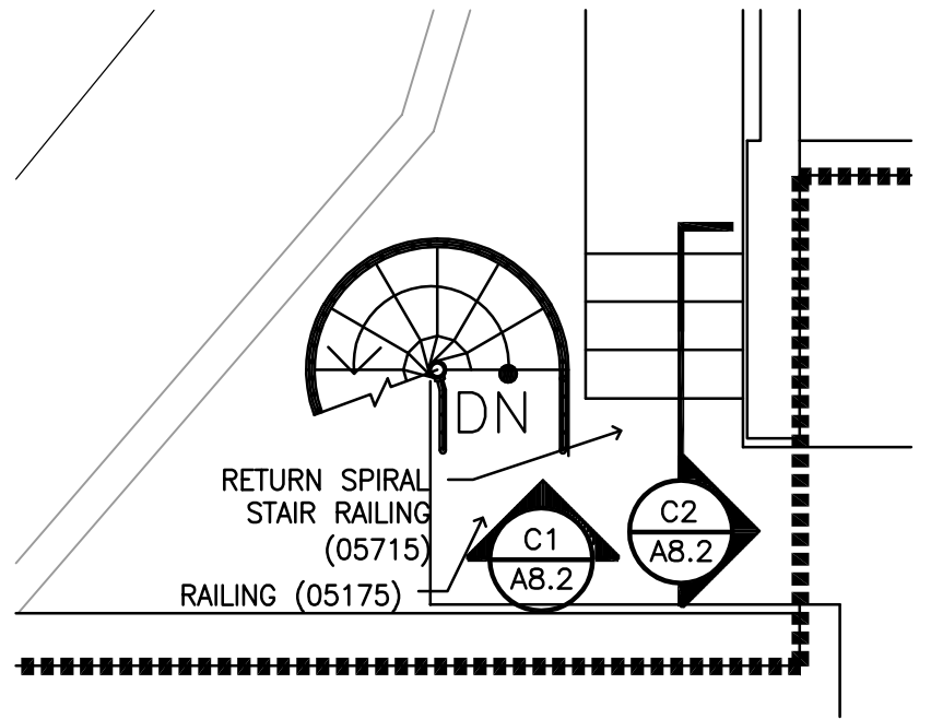
A2 SPIRAL STAIR 'B' - TOP A8.2 1/4"=1'-0"
