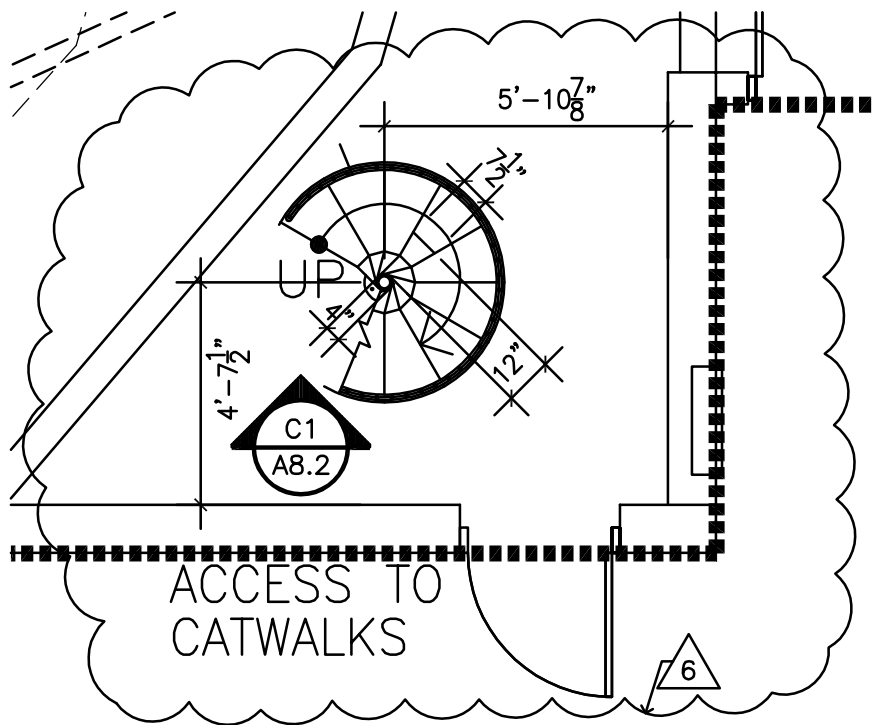
A1 SPIRAL STAIR 'B' BASE A8.2 1/4"=1'-0"
