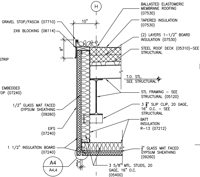
A4 A4.4 EIFS DETAIL 3" = 1'-0"
